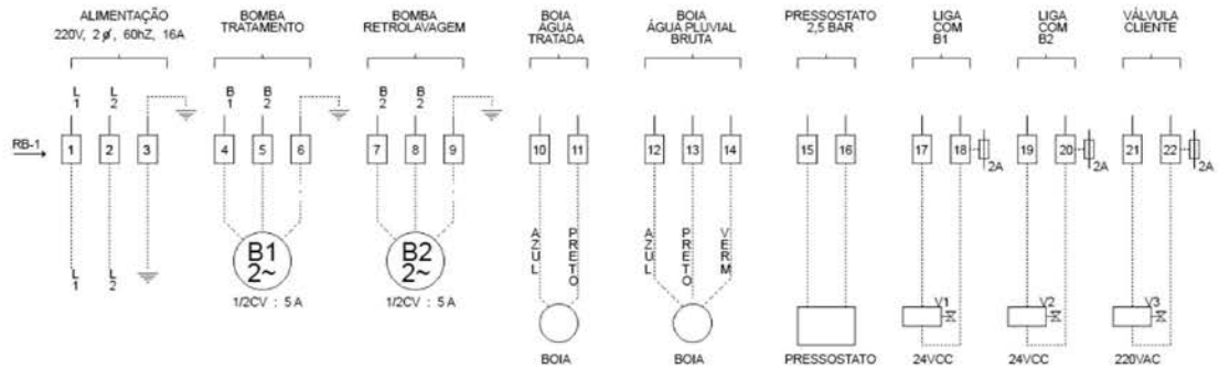
Figura 04 – Ligação dos bornes
