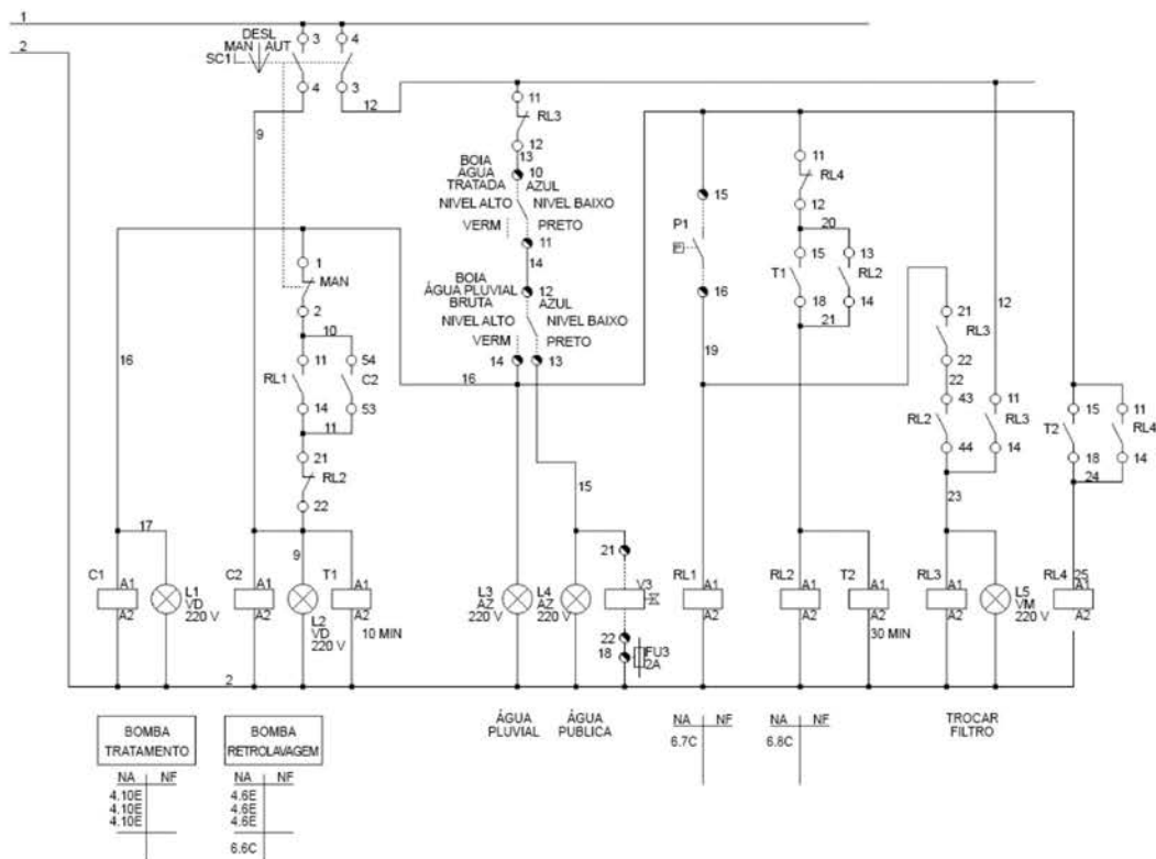
Figura 06 – Diagrama de comando
