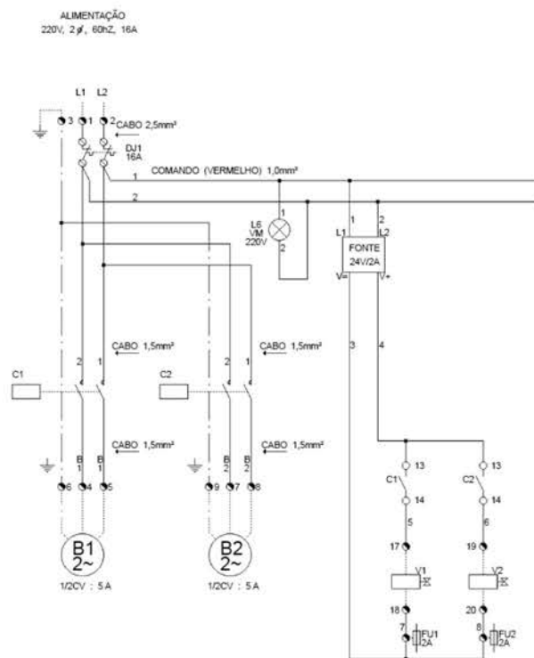
Figura 05 – Diagrama de potência
